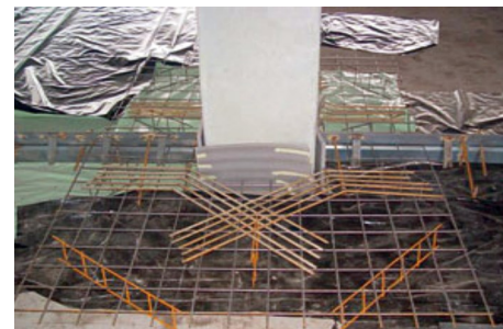
Obr. 4: Obvodová dilatácia podlahy v mieste stĺpa
