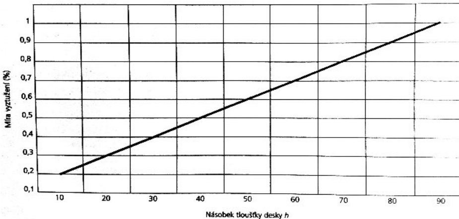
Obr. 5: Vzdialenosť kontrakčných škár ako funkcia stupňa vystuženia [4]
