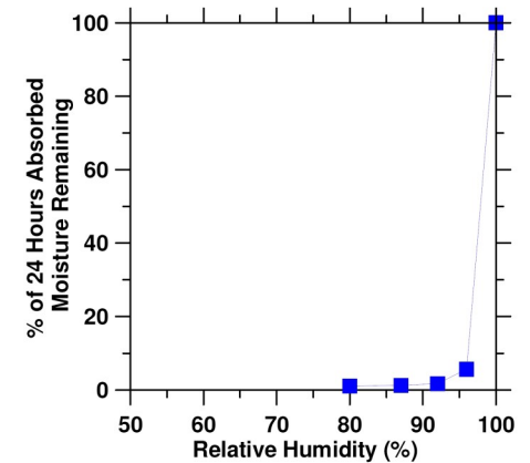
Obr. 3: Desorpčná krivka SLWA [10]
