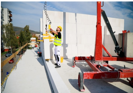
Obr. 3: Ytong Jumbo, práca s minižeriavom
