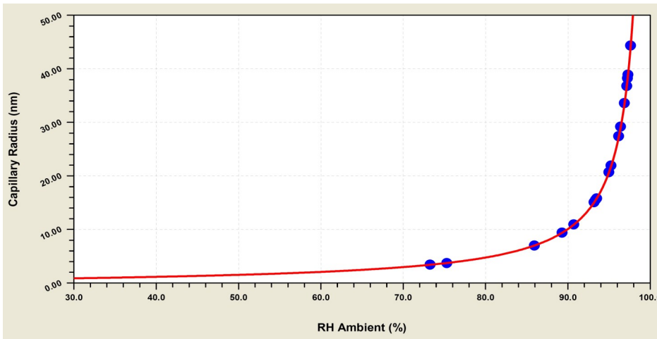
Obr. 2: Polomer kapilár ako funkcia RH
