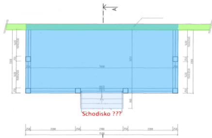
Obr. 3: Pôdorys skleníka
