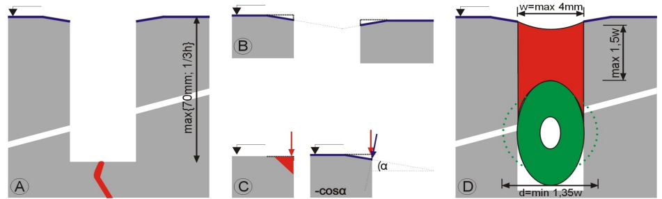
Obr. 11: Úprava a výplň rezanej škáry (A – úprava zbrúsením hrán; B – pokles platní pri zaťažení a vytvorenie nábehu; C – zníženie šmykového zaťaženia hrany; D – zásady vyplňovania škár)
