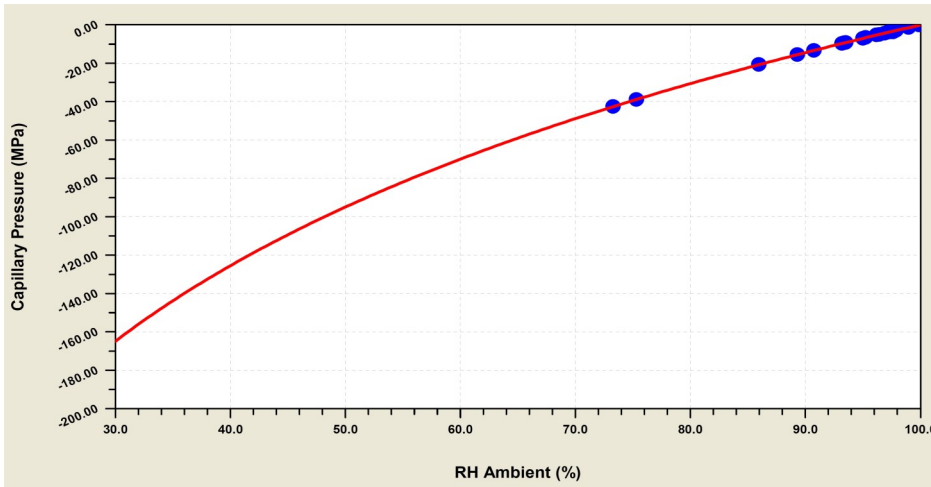
Obr. 1: Kapilárne napätie ako funkcia RH
