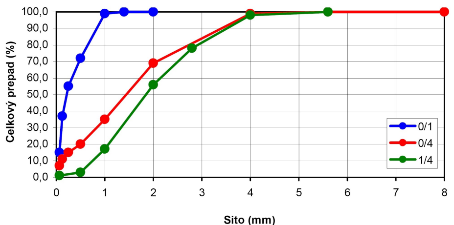
Obr. 8: Čiary zrnitosti skúšobných frakcií
