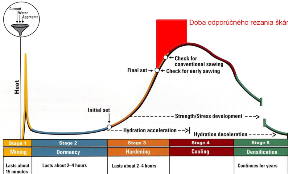
Obr. 9: Vhodná doba pre rezanie škár [5]
